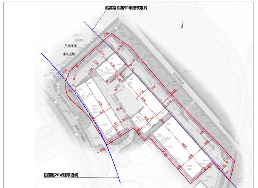
退线退距图
